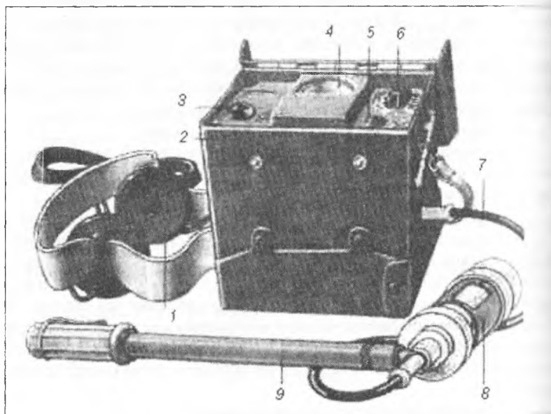
Рис. 66. Измеритель мощности дозы (рентгенметр) ДП-5В:
