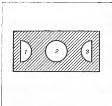
Рис. 25. Фазы Луны: 1 — первая четверть; 2 — полнолуние; 3 — последняя четверть
